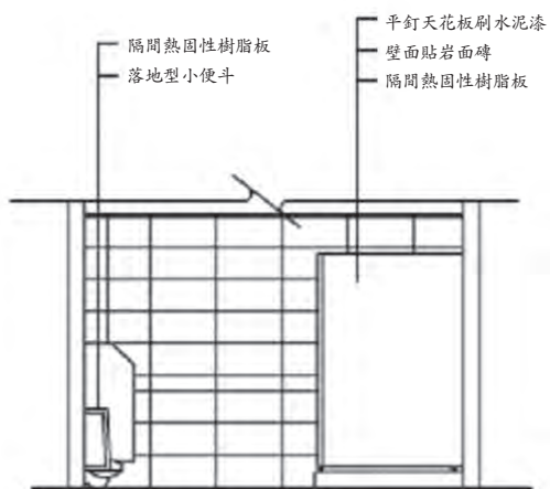
施工設計圖
