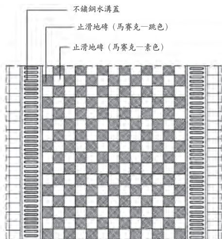
施工設計圖
