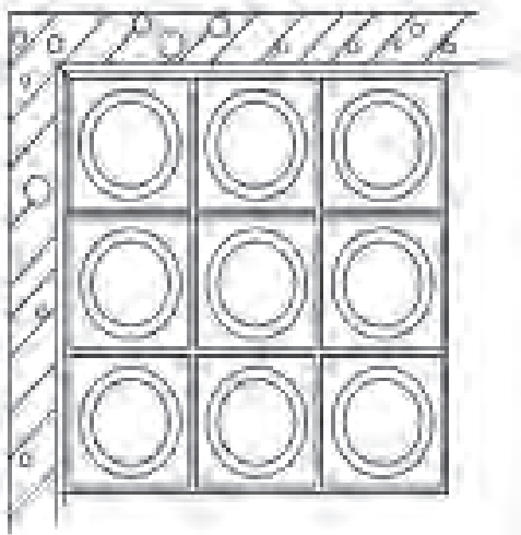
施工設計圖
