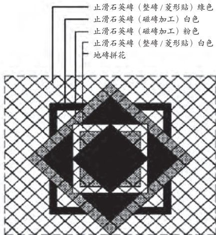
設計示意圖
