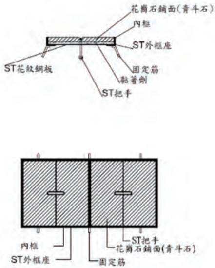
設計示意圖
