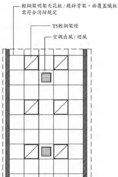
設計示意圖
