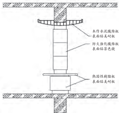
施工設計圖
