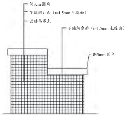
施工設計圖
