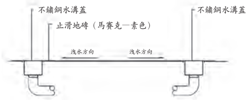
施工設計圖
