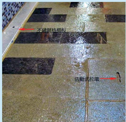
水溝蓋板下方設計不銹鋼洩水孔板，溝渠不阻塞。
