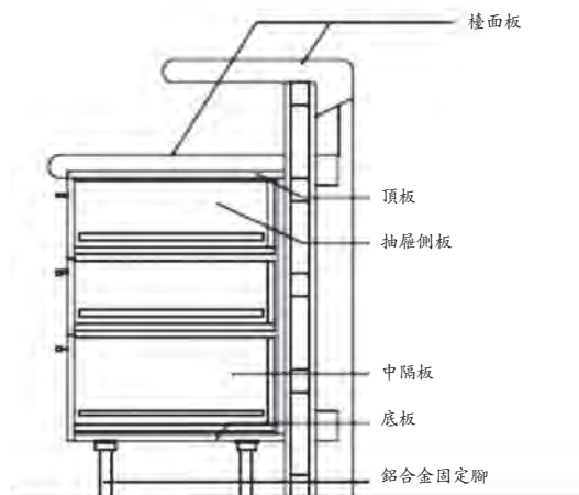
施工設計圖
