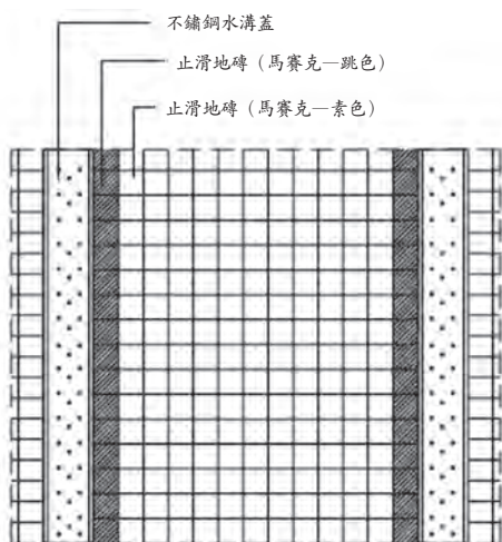
施工設計圖
