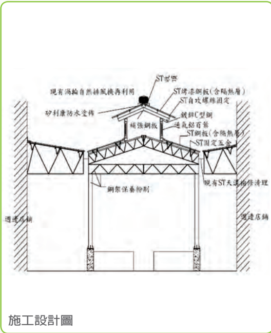
太子樓屋頂 + 鏤空頂板鐵網架通風性佳
